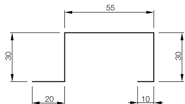
C1SRP Hřebenový/náročný profil nevětraný, dl. 2000 mm
