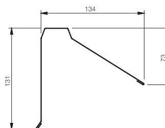
OVKSRP Přechodový plech – vikýře, dl. 2000 mm
