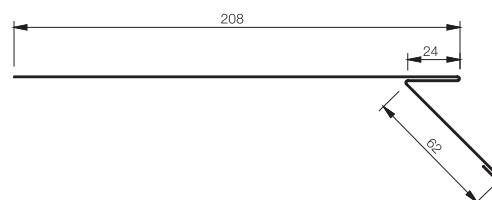
FSRP Zatahovací okapový plech, dl. 2000 mm
