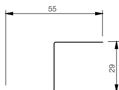
C2SRP Napojovací lišta, dl. 2000 mm
