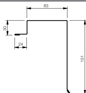
VISRP Závětrná lišta- vrchní, dl. 2000 mm
