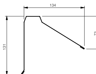
OVKSRP Přechodový plech – přechod sklonů, dl. 2000 mm
