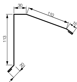
VISK-S – závětrná lišta pro taškovou krytinu – spodní, dl. 2000 mm
