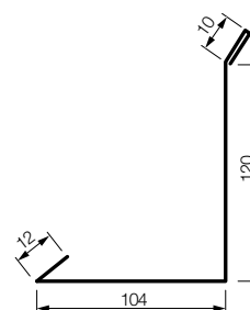
VISK-GL – závětrná lišta pro krytinu GOODLOCK, dl. 2000 mm
