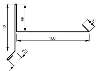
VISK-S – závětrná lišta pro taškovou krytinu – spodní, dl. 2000 mm
