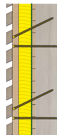
Schéma pro upevnění tepelné izolace na stěny. Vrty jsou namáhány na tah a na tlak.
